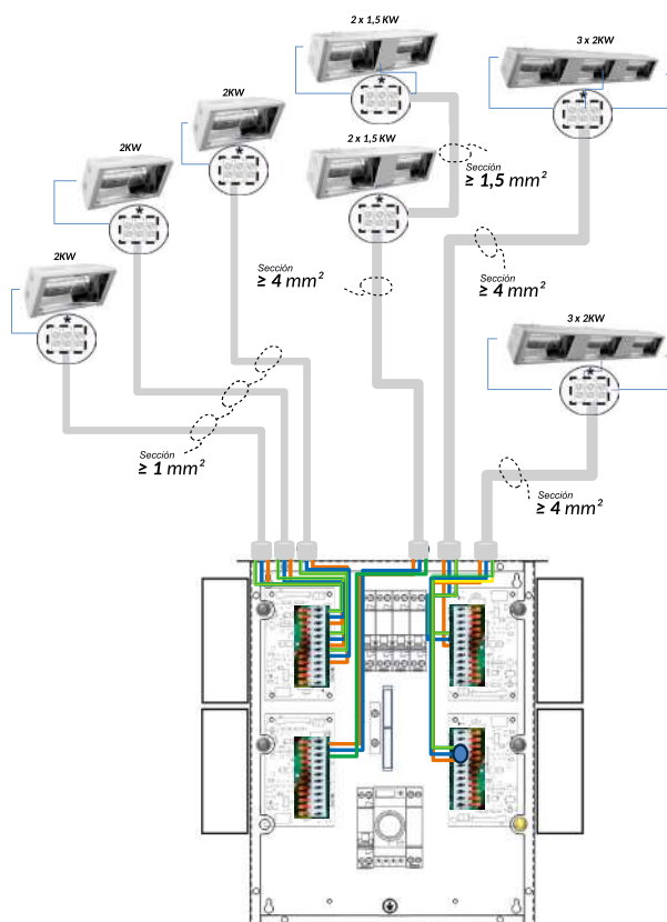
ESQUEMA DE CONEXIONES STAR24
