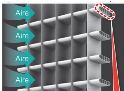
Intercambiador de tubos planos
