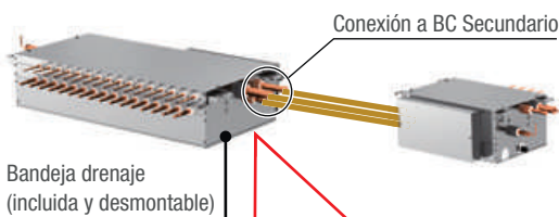
Modelo actual (CMB-M V-JA1/KB1, CMB-P V-KA1)
