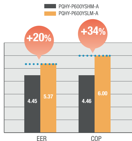
-Comparativa de un módulo combinado (300+300)
