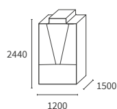
RHMA 18AN RHMA 24AN (Versión con bomba fija o sin bomba)
