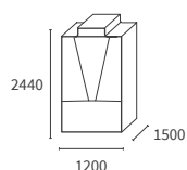
RHMA 18AX RHMA 24AX (Versión con kit de bomba de velocidad fija o sin kit de bomba)
