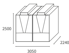
RHMA 60AN RHMA 75AN RHMA 90AN RHMA 100AN (Versión con bomba variable o sin bomba)
