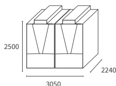
RHMA 60AX RHMA 75AX RHMA 90AX RHMA 100AX (Versión con kit de bomba de velocidad variable o sin kit de bomba)
